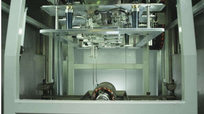
Träufelmodul der bdtronic Imprägnieranlage.
